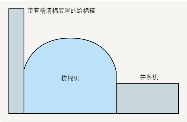
图36 组合梳棉机
