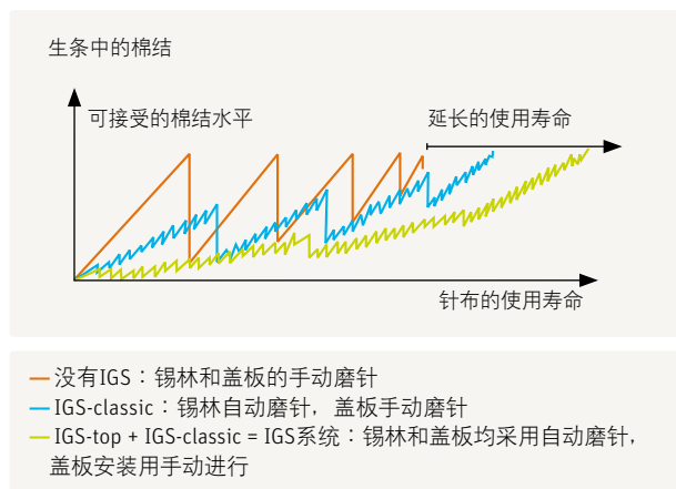
图146 使用IGS系统带来的质量提高
