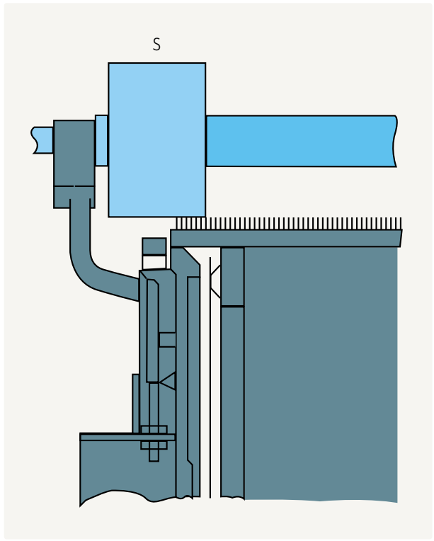
图138 横向运动的研磨圆盘
