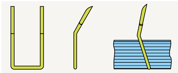
图120 弹性针布
