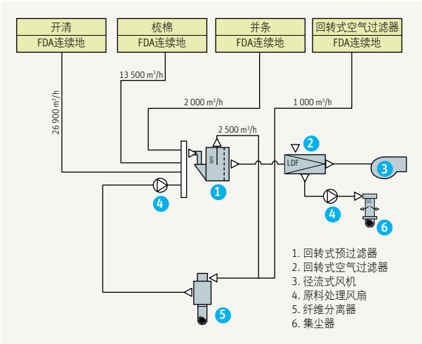
图83 除尘流程图
