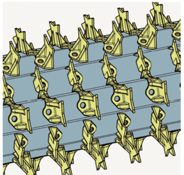
图39 开松装置
