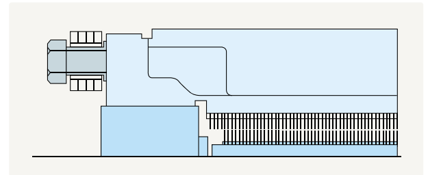
图110 通过螺丝将盖板条固定在环状链条上
