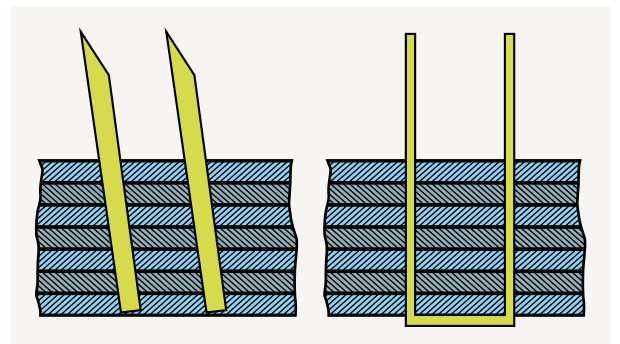
图121 半硬性针布
