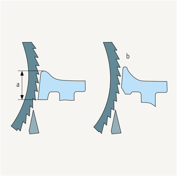
图96 给棉板的形状
