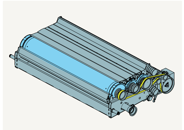
图140 刺辊模块
