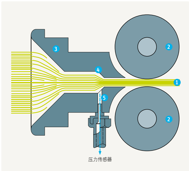
图133 积极式气动测量系统（Zellweger, Uster）
