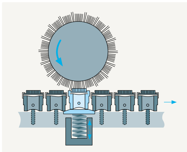
图145 盖板自动磨针系统IGS-top
