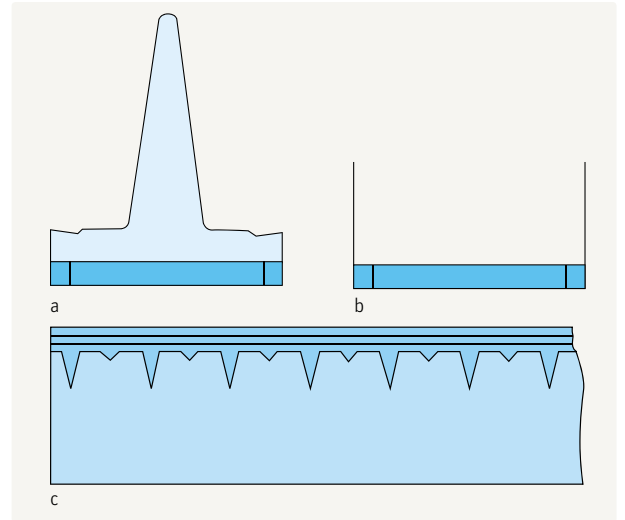
图108 使用边夹（c）将针布条（b）安装在盖板条（a）上
