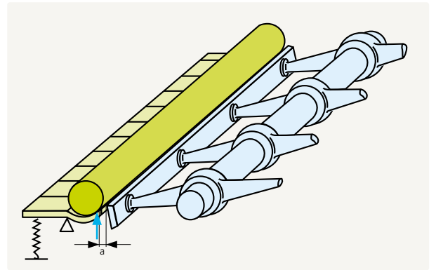
图12 通过一个给棉罗拉和天平杆将原料喂入打手
