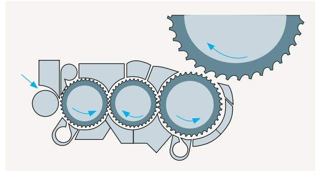
图101 立达三刺辊梳棉机C 60
