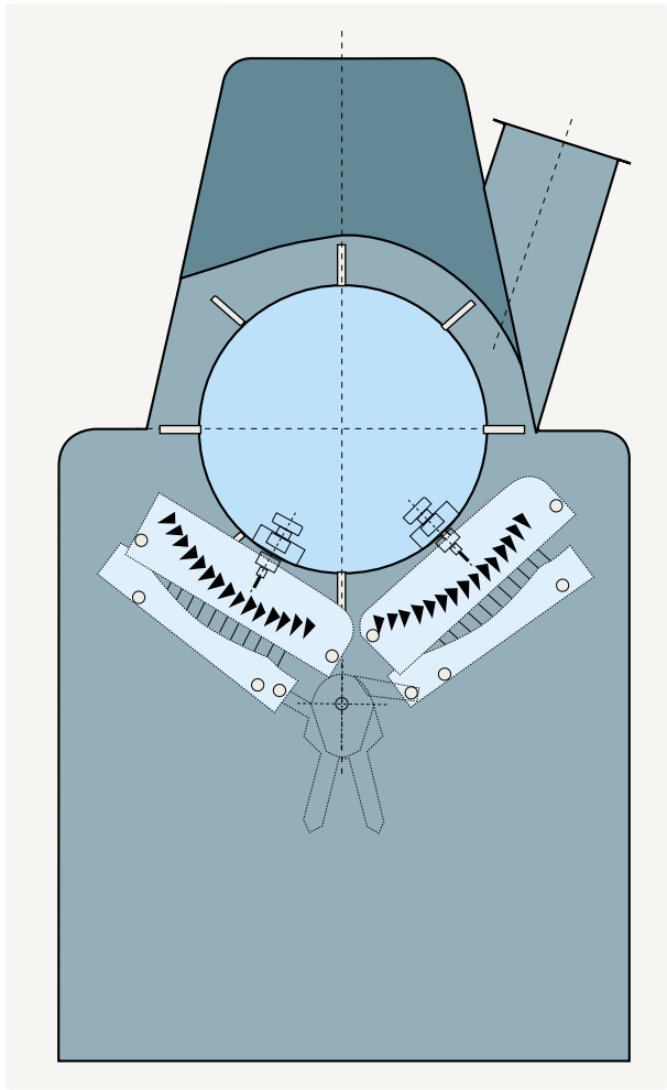
图25 两部分尘格
