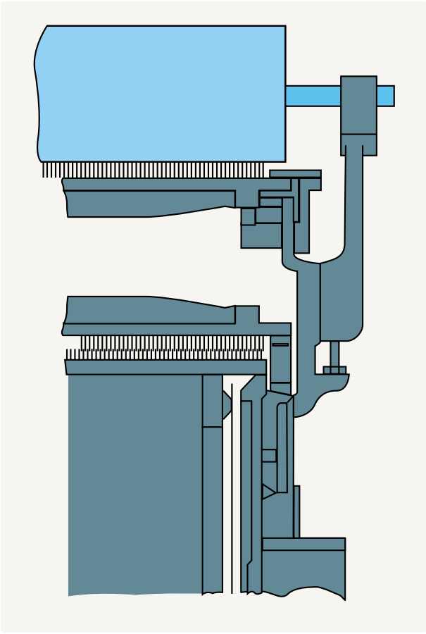
图137 研磨辊
